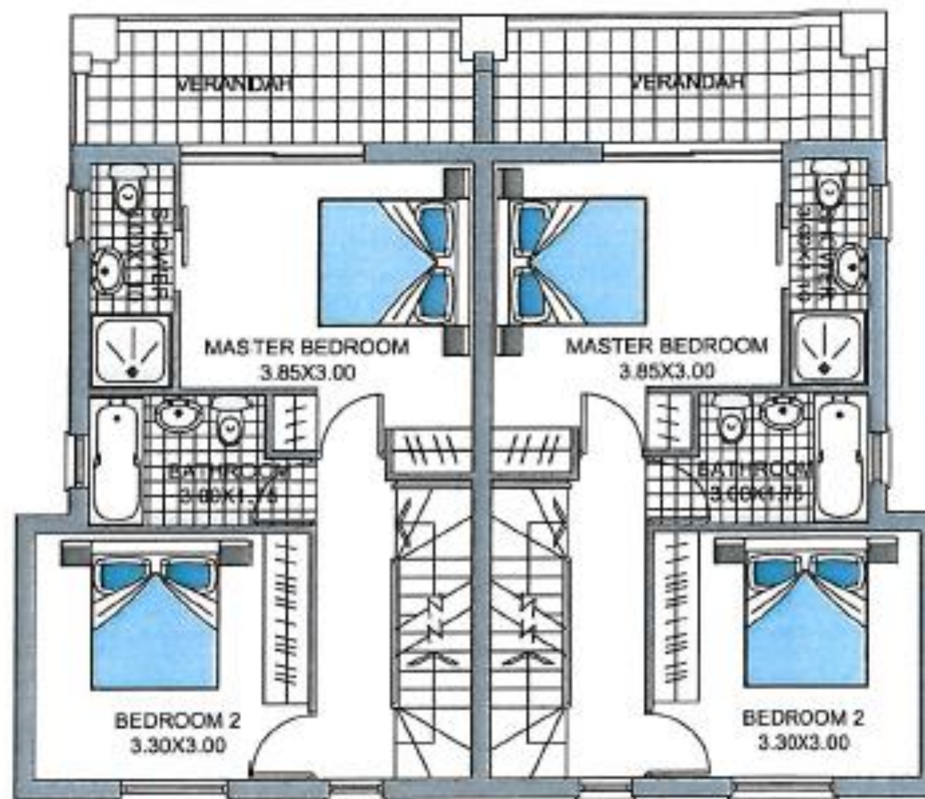
ВТОРОЙ ЭТАЖ
